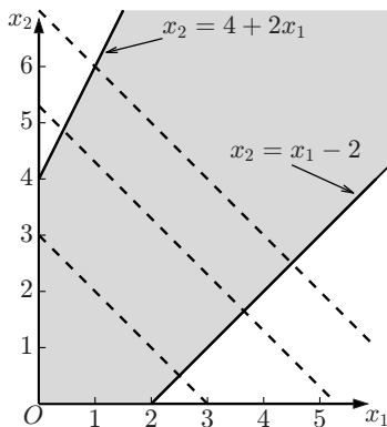
图 2.4 无界解
